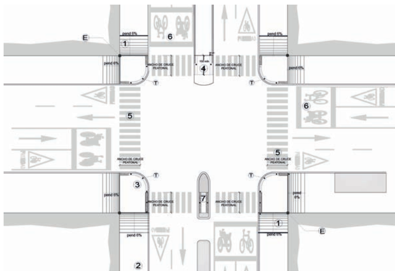
Planta: intersección
