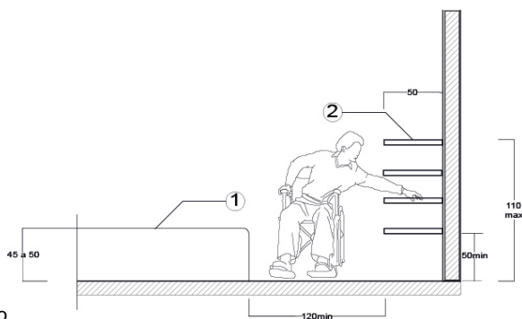
Alzado
