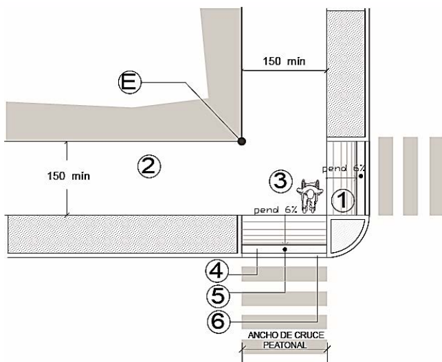
Planta: variante 1
