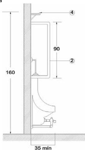
Alzado lateral
