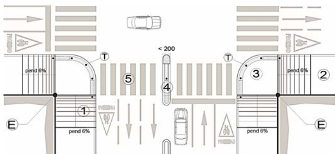
Planta: variante 1
