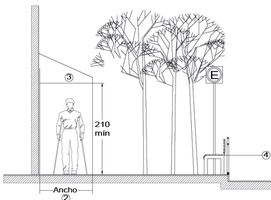
Alzado frontal
