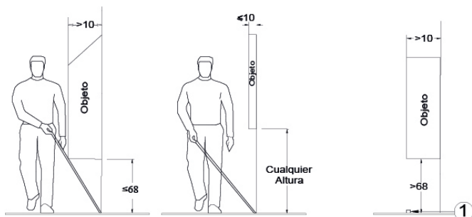
Alzado frontal
