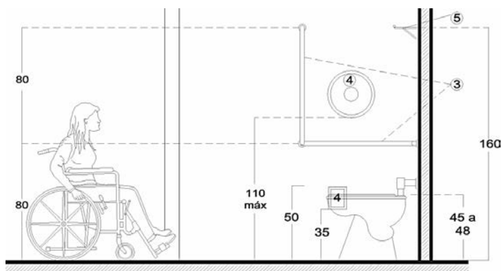
Alzado
