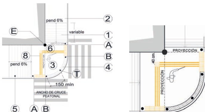
Plantas: variante 2.
