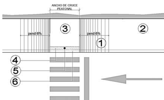
Planta: variante 2
