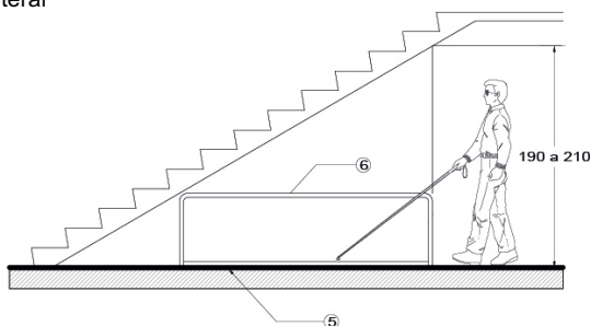
Alzado lateral
