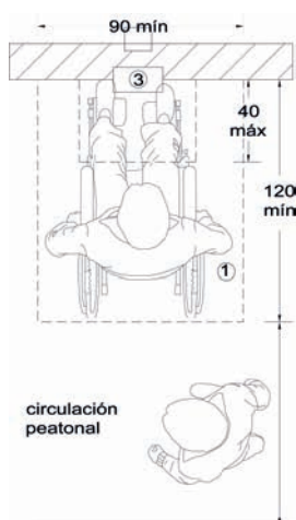
Planta
