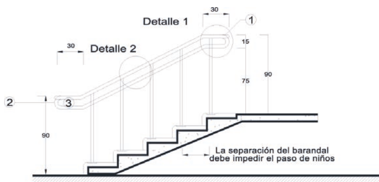
Alzado lateral
