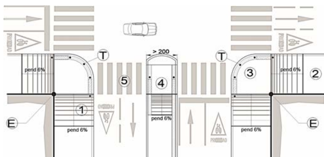
Planta: variante 2
