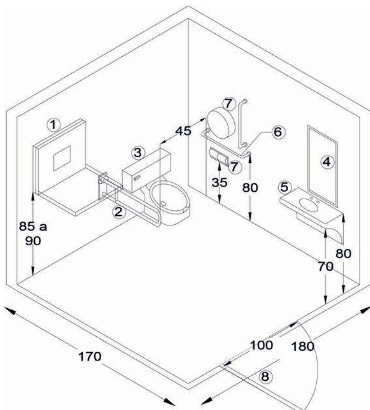
Isométrico
