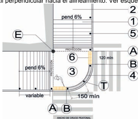
Planta: variante 1.
