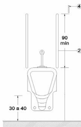
Alzado frontal
